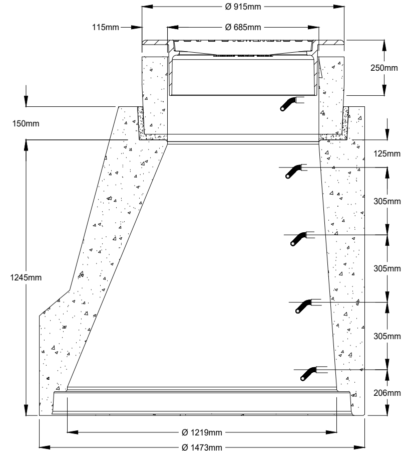
SECTION A-A
